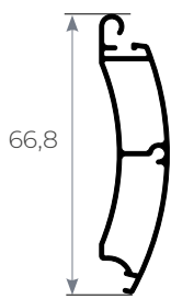
PROFILO LAMELLA
