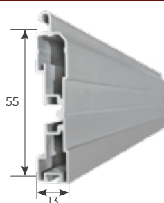
VARIANTE Terminale 13x55 in alluminio estruso
