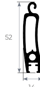
STECCA SUPERIORE
