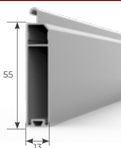
STANDARD Terminale 13x55 in alluminio estruso standard
