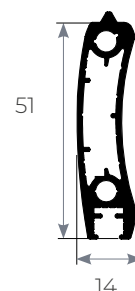
PROFILO LAMELLA
